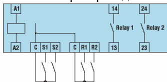
Трехпроводная схема управления
