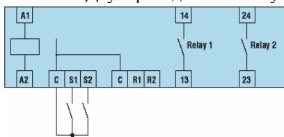
Двухпроводной схемы управления
